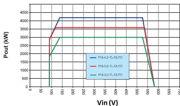
Pout Vs Vin (double input channel)
