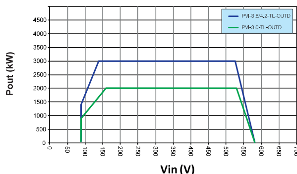
Pout Vs Vin (single input channel)
